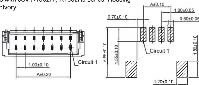
P.C.B LAYOUT
