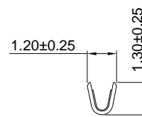
SEC:B-B
