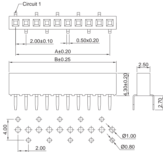
P.C.B LAYOUT
