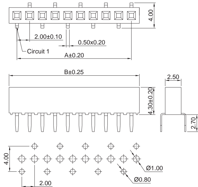
P.C.B LAYOUT
