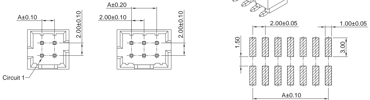
P.C.B LAYOUT
