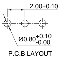
P.C.B LAYOUT
