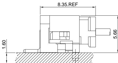
SMT TYPE
